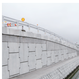
補強土壁(テールアルメ)
