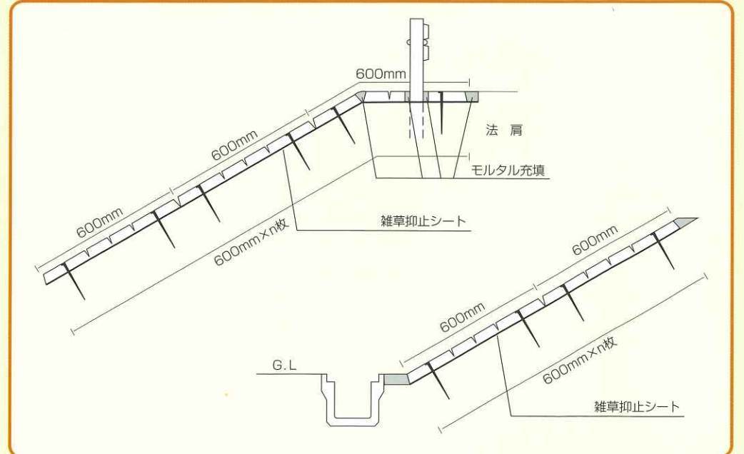
抜け止め加工品納まりイメージ
