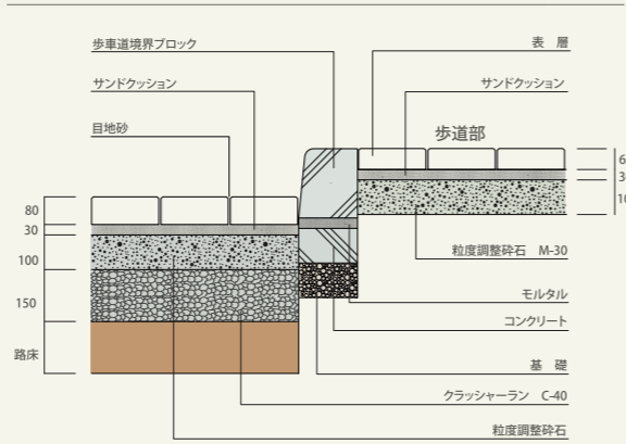
■縁石をインターロッキング面にあわせる場合
