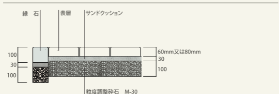
■縁石をインターロッキング面にあわせる場合
